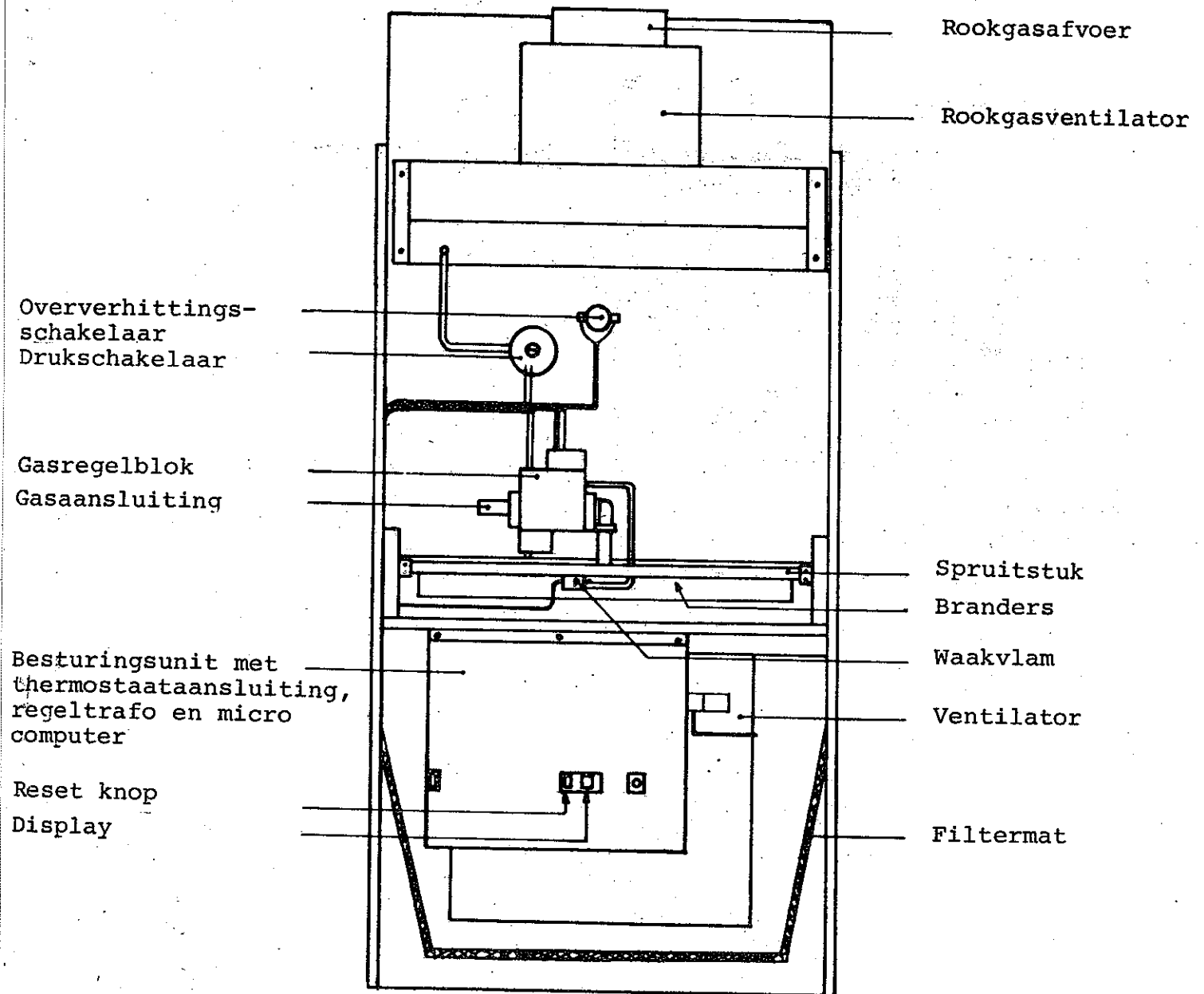
1 Figuur 6 :Vooraanzicht luchtverwarmer type H met bedieningsapparatuur.
