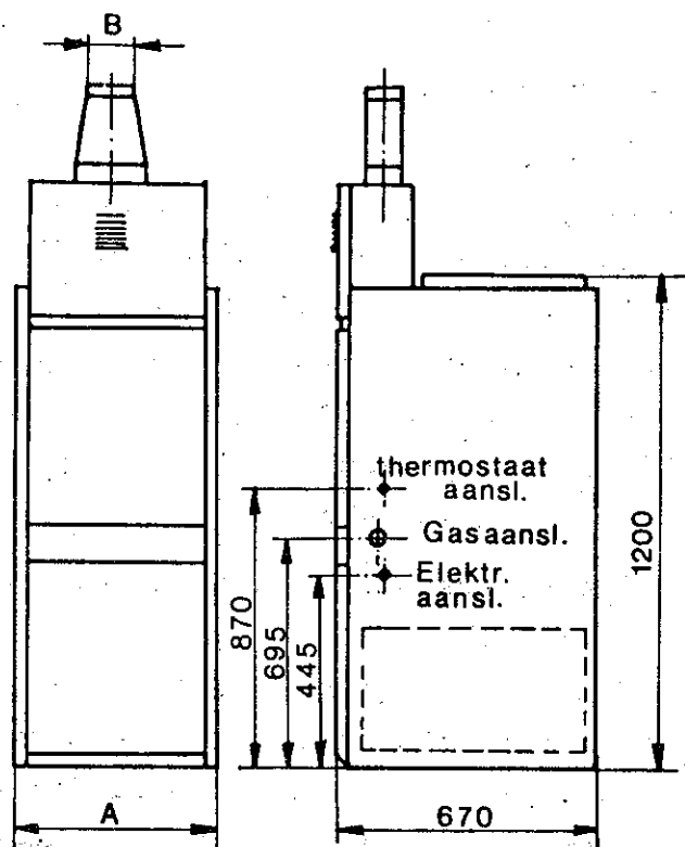
Figuur 5. Aansluitpunten luchtverhitter.
