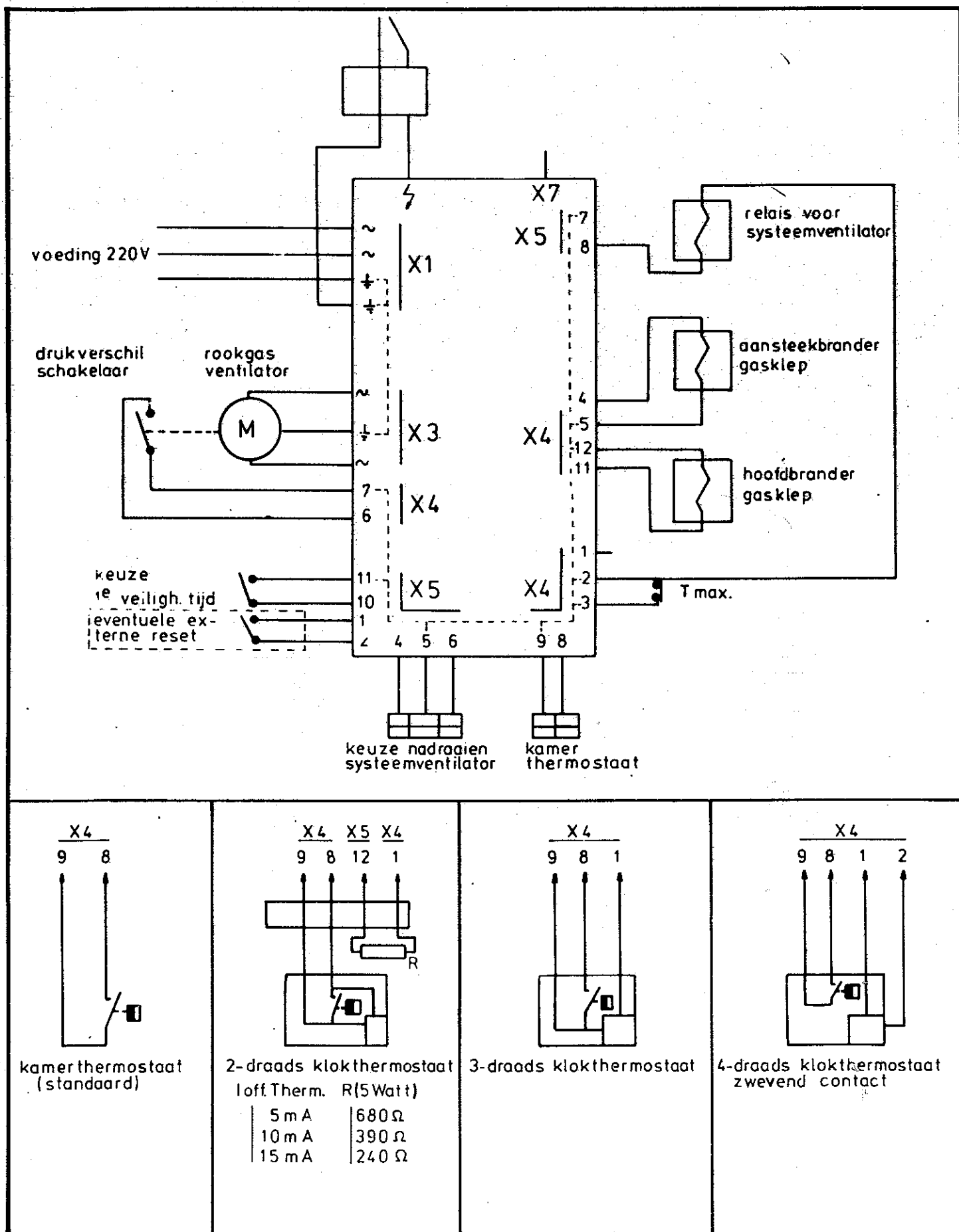
Fig. 9 : Aansluitschema besturingskast Philips MCBA 0211.
